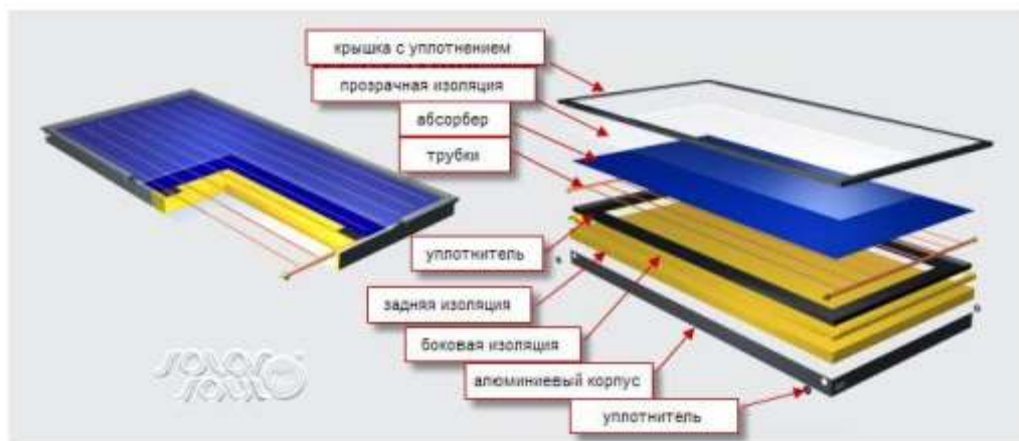
Рис.1 Плоский солнечный воздухонагреватель
