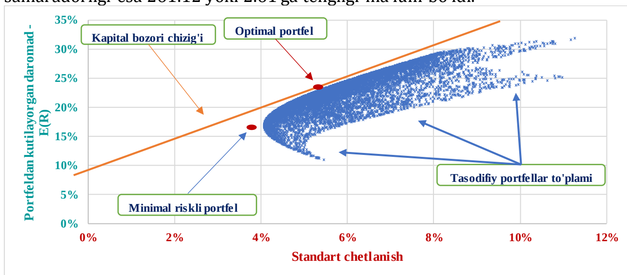
1-rasm. Monte-Karlo simulatsiya usuli asosida shakllantirilgan tasodifiy portfellar
