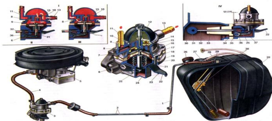
2-rasm. Yonilg'i nasosi, filtrlar, yonuvchi aralashmasining xususiyatlari
