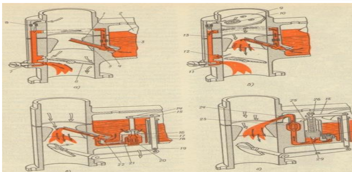
4-rasm. Karbyuratorning tuzilmalari: A-aralashmani kompensatsiyalash tuzilmasi; B-salt ishlash tuzilmasi; V-tezlatgich tuzilmasi; D-yurgizib yuborish tuzilmasi.
