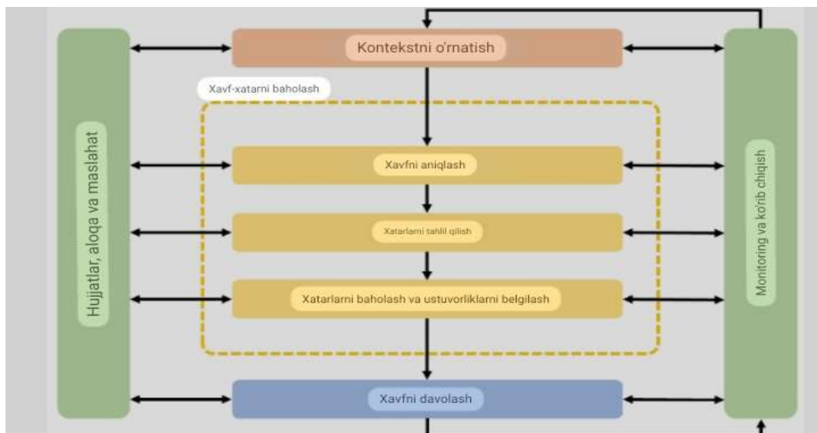
1-rasm. Bojxona tizimida risklarni boshqarish tizimi
