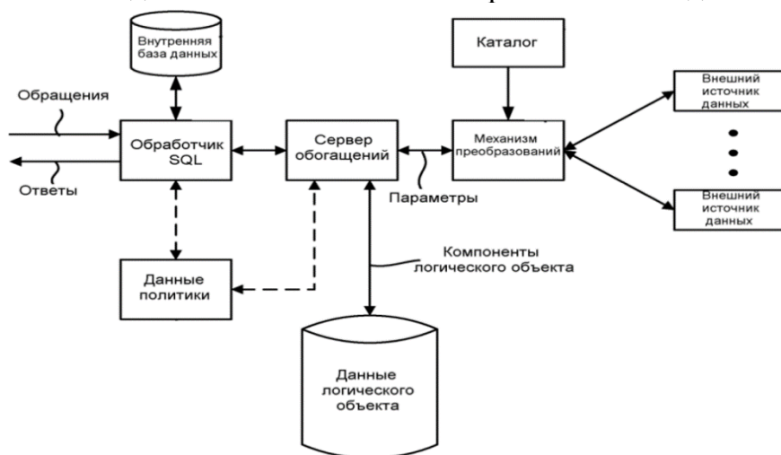
Рисунок 1. Схема структурного процесса запроса чётных форм.
