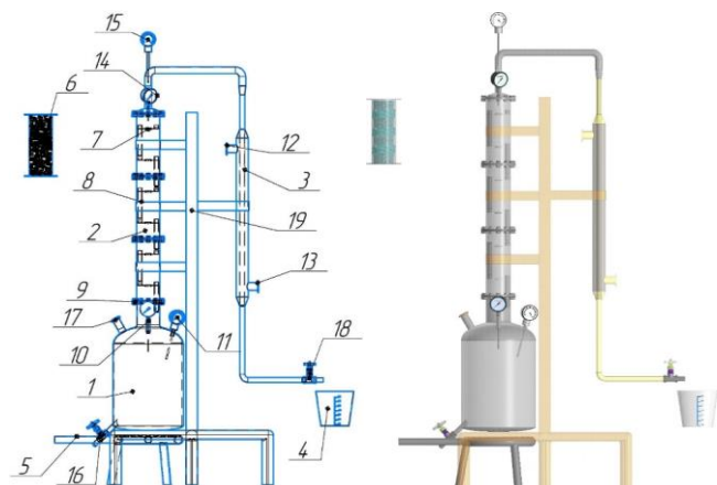
Рис. 2 – Установка для изучения процесса ректификации многокомпонентных углеводородных смесей.
