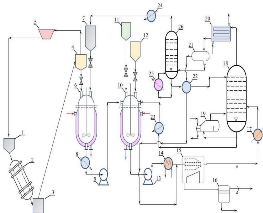
1-rasm. Polipropilen asosli dizel yoqilg'isining quyi haroratdagi xossalarini yaxshilovchi prisadkalarni olishning uzluksiz prinsipial texnologik sxemasi
