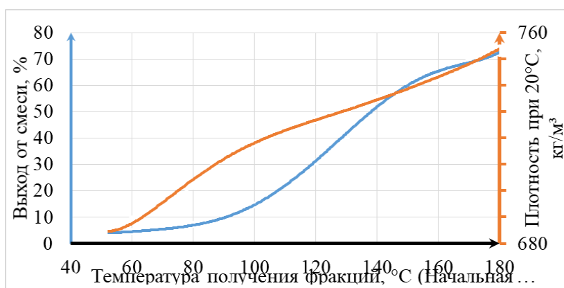
Рис. 4. Зависимость выхода и плотности бензиновой фракции от температуры
