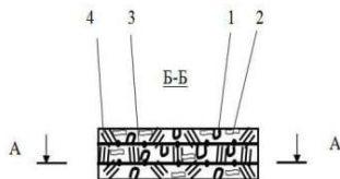
1-súwret. Boylama kesimdegi órtke shıdamlı gerbish. 1-tiykarǵı órtke shıdamlı elementtiń bólekleri, 2-baylanıstırıwshı, 3-joqarı temperaturalı uglerod talshıǵınan jasalǵan bekkemlewshi tor, 4-kesilgen oralǵan joqarı temperaturalı uglerod talshıǵınan jasalǵan keńislikke baǵdarlanǵan talshıqlar.
