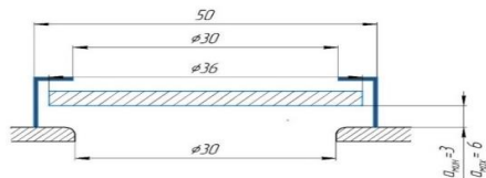
Рис. 1. Сравнительная конструкция элементов колонн: клапанная тарелка и спирально-призматическая насадка 20х30.
