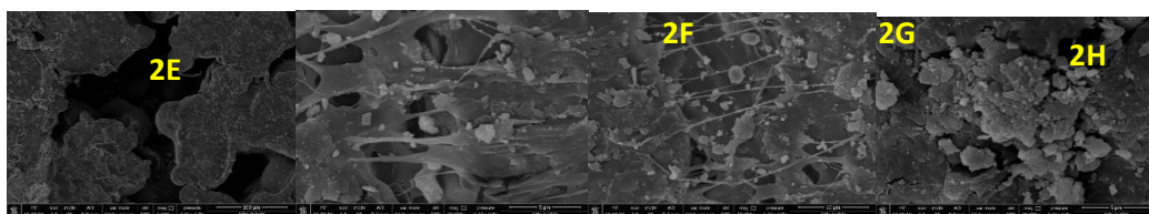
2-rasm. PLA/HA 80:20 tarkibli hamda namuna massasiga nisbatan 10% miqdorda Mg_3(PO_4)_2 modifikator qo'shishdan olingan materiallar SEM analizi natijalari
