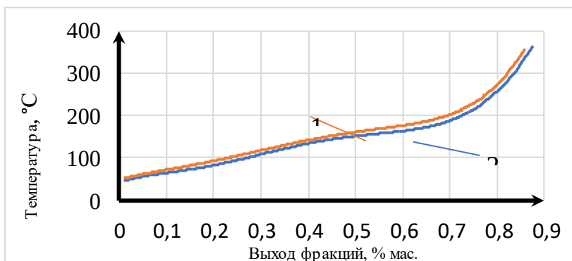
Рис. 3. Итоги экспериментов по изучению фракционного состава смеси нефтегазоконденсата (30% нефти и 70% газоконденсата), проведенных с использованием насадочно-клапанной колонны (2) и клапанной колонны (1).
